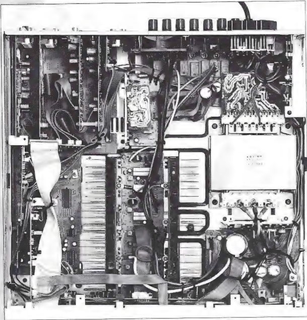
Het interieur van de VSA-E06
